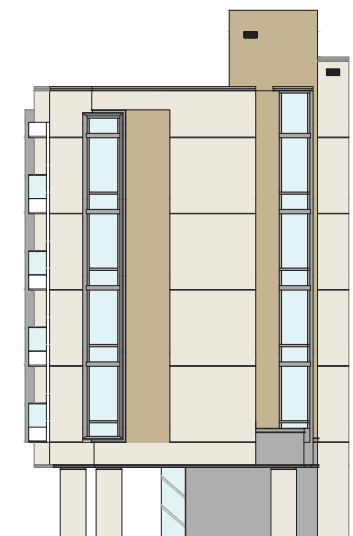
ELEVATION PLAN 14 立面圖 14
